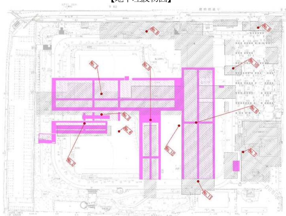
【地下埋設物図】
